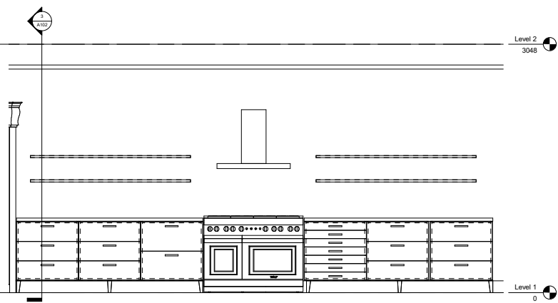
4 Section 3 1 : 20
