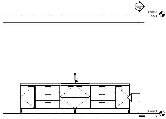
2 Section 1 1 : 20
