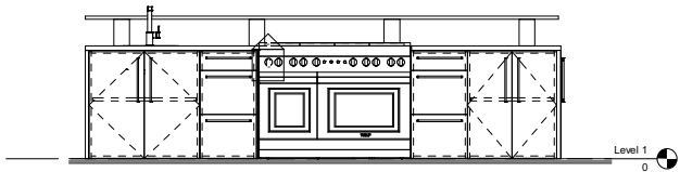
② Section 1 1 : 20
