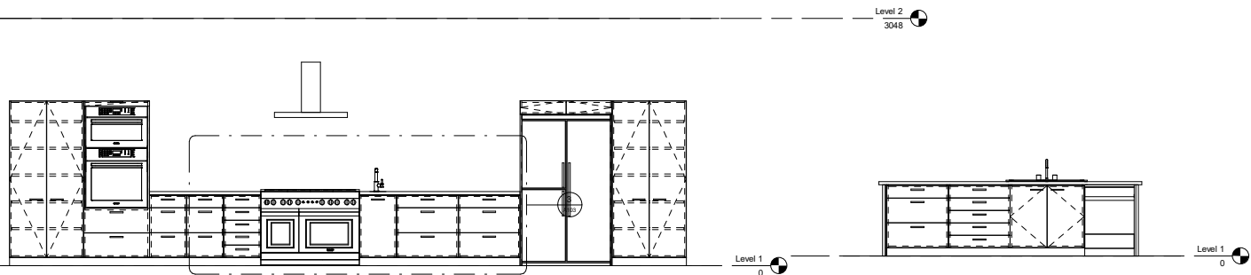
① Section 1 1:25
