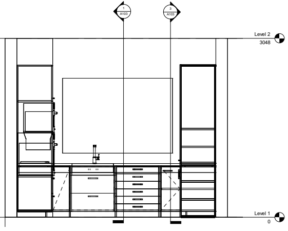
② Section 2 1 : 20
