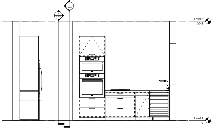
① Section 1 1 : 20
